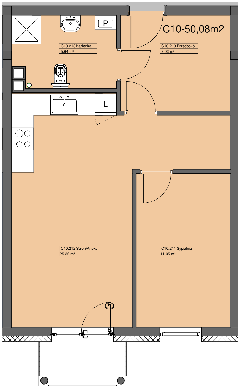
1 Rzut I Piętra — Lokal C10 1 : 50
