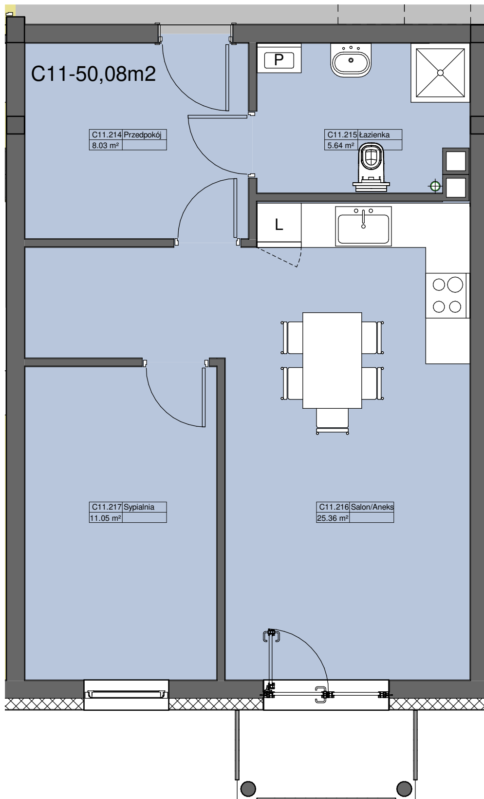
1 Rzut I Piętra — Lokal C11 1 : 50
