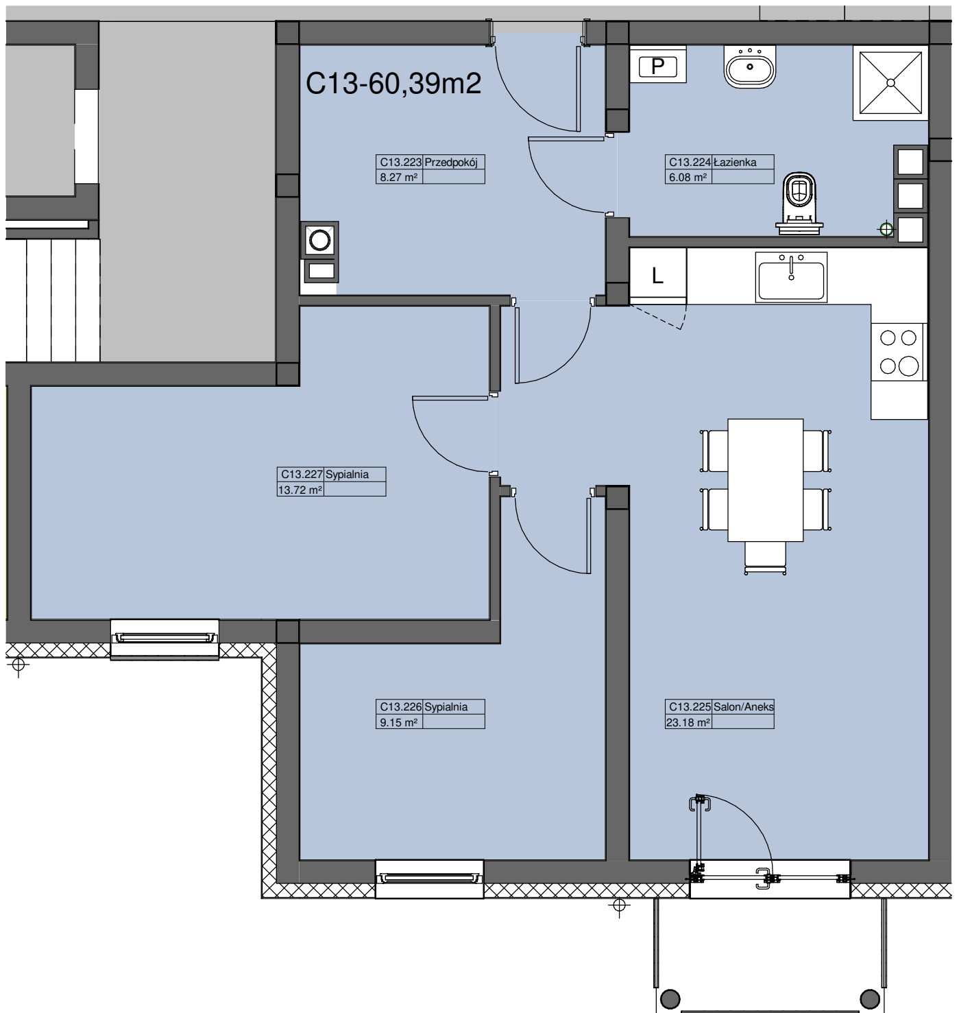
1 Rzut I Piętra — Lokal C13 1 : 55
