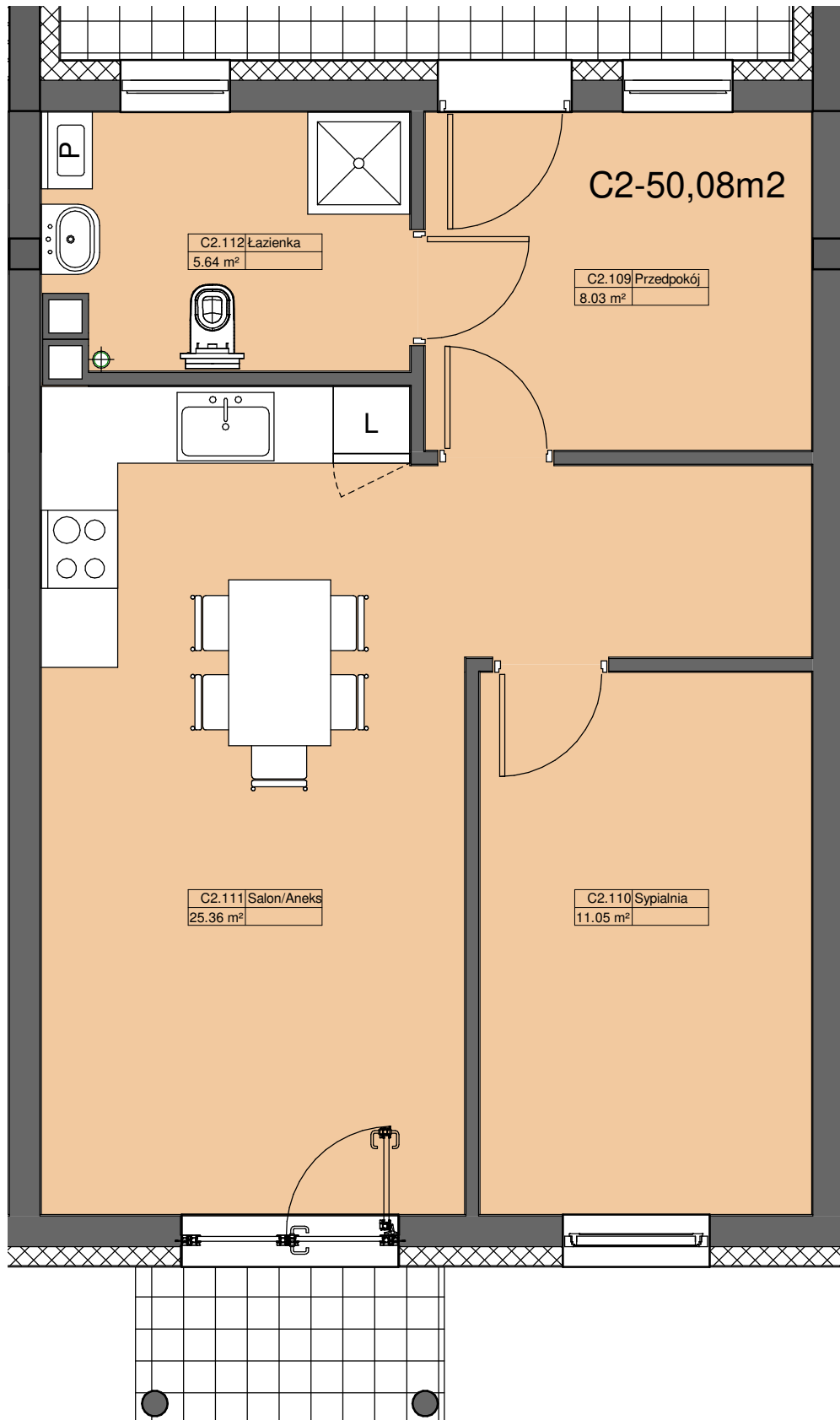
1 Rzut Parteru — Lokal C2 1 : 50
