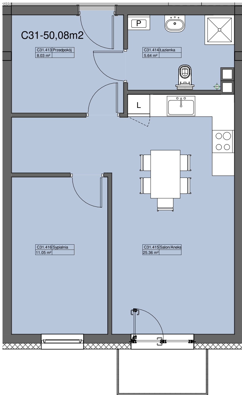
1 Rzut Poddasza — Lokal C31 1 : 50
