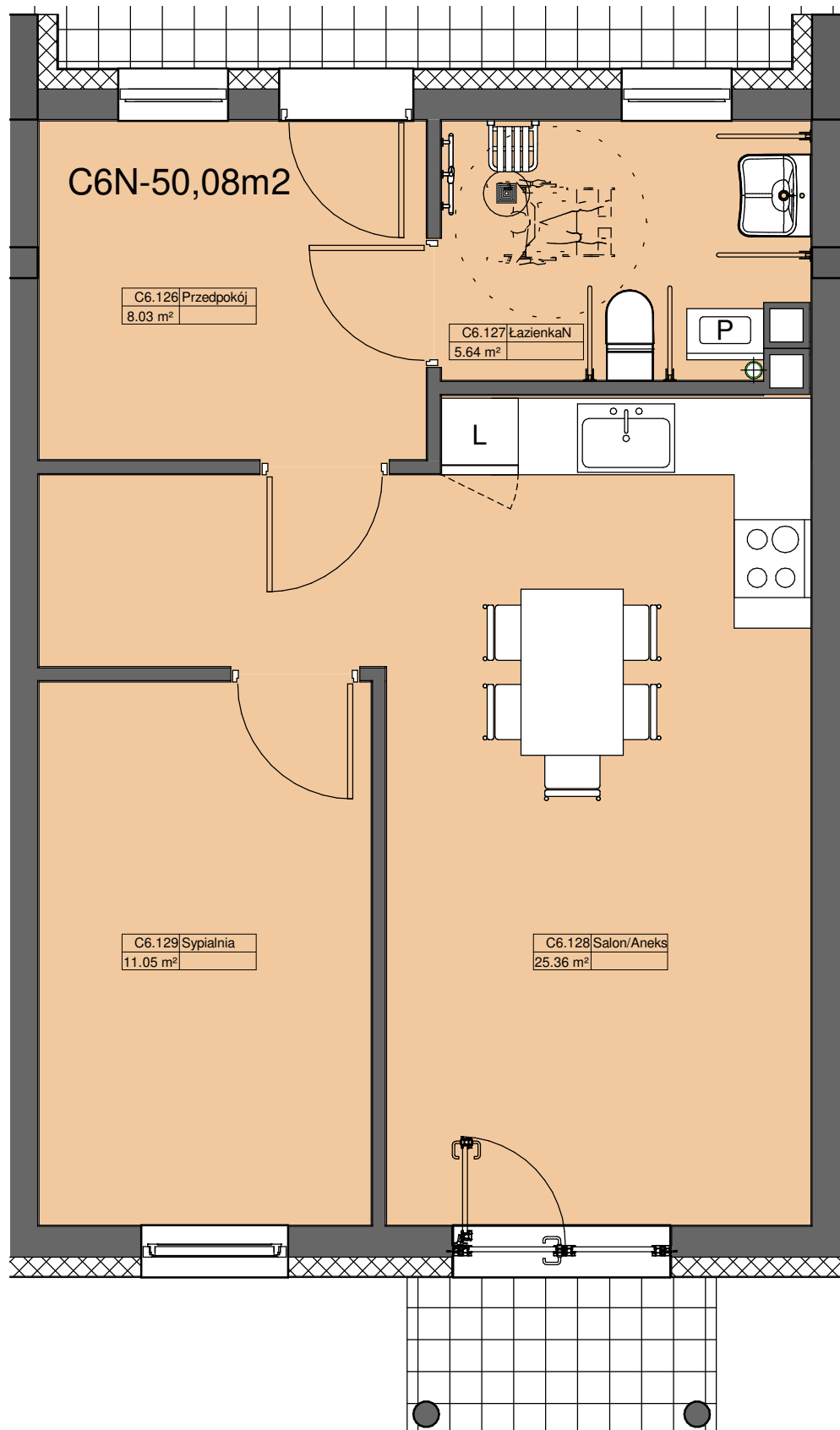
1 Rzut Parteru — Lokal C6 1 : 50
