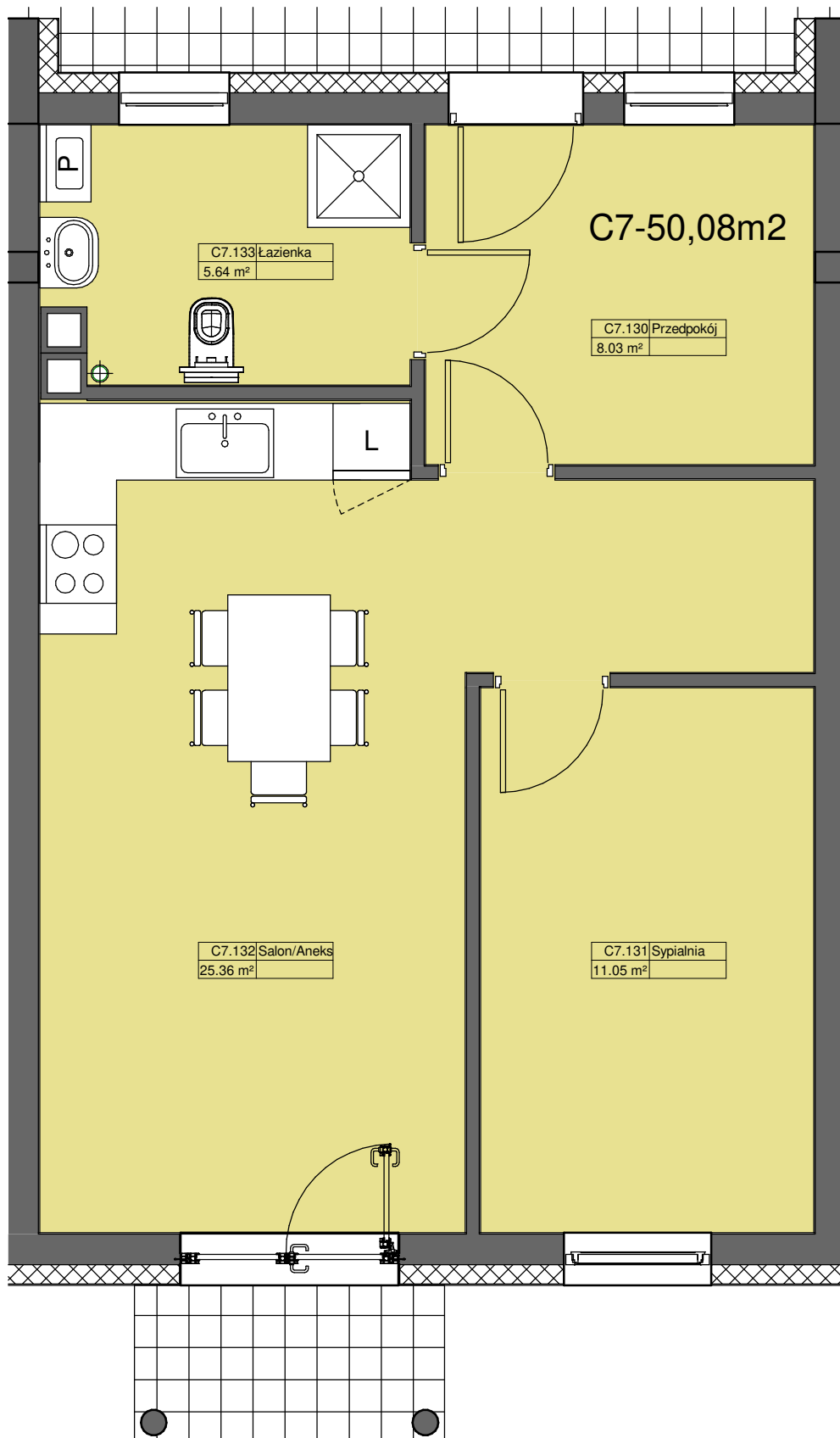
1 Rzut Parteru — Lokal C7 1 : 50
