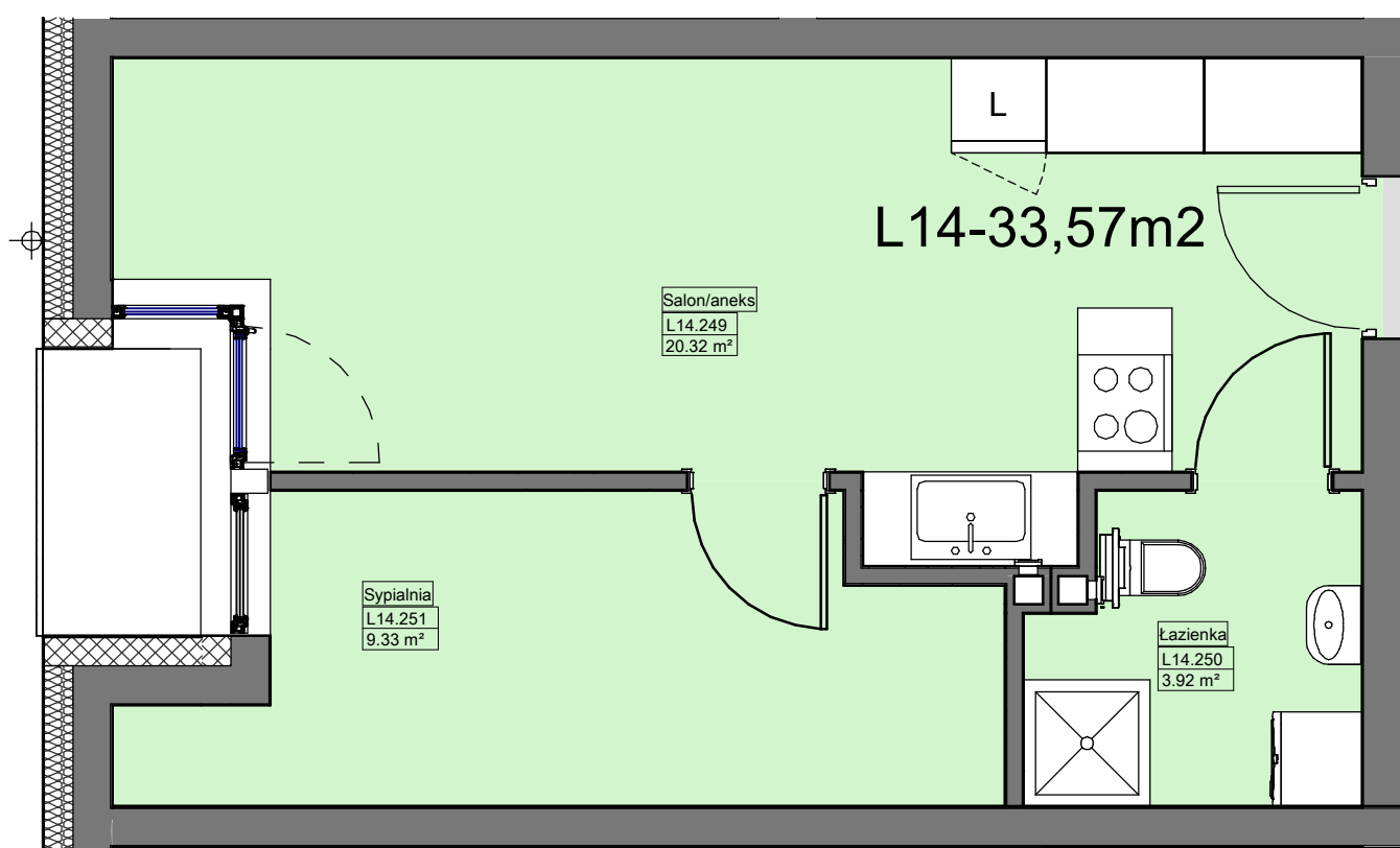
1 Rzut I Piętra — Lokal L14 1 : 50
