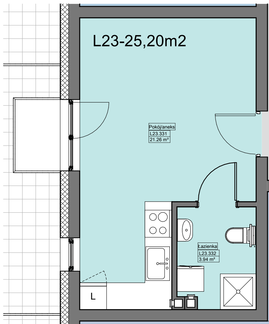
1 Rzut II Piętra — Lokal L23 1 : 50
