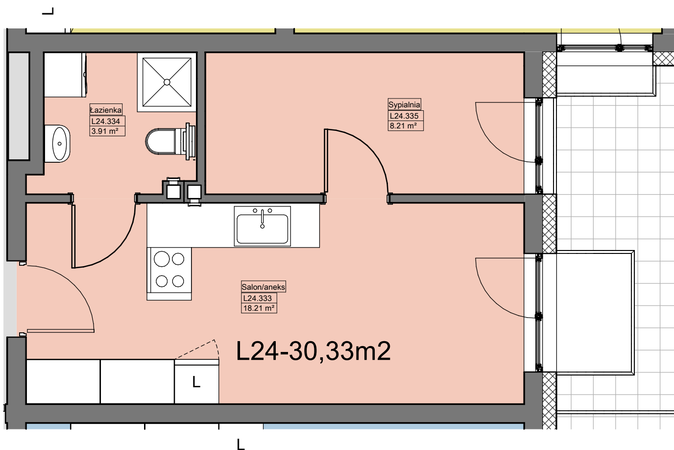
1 Rzut II Piętra — Lokal L24 1 : 50
