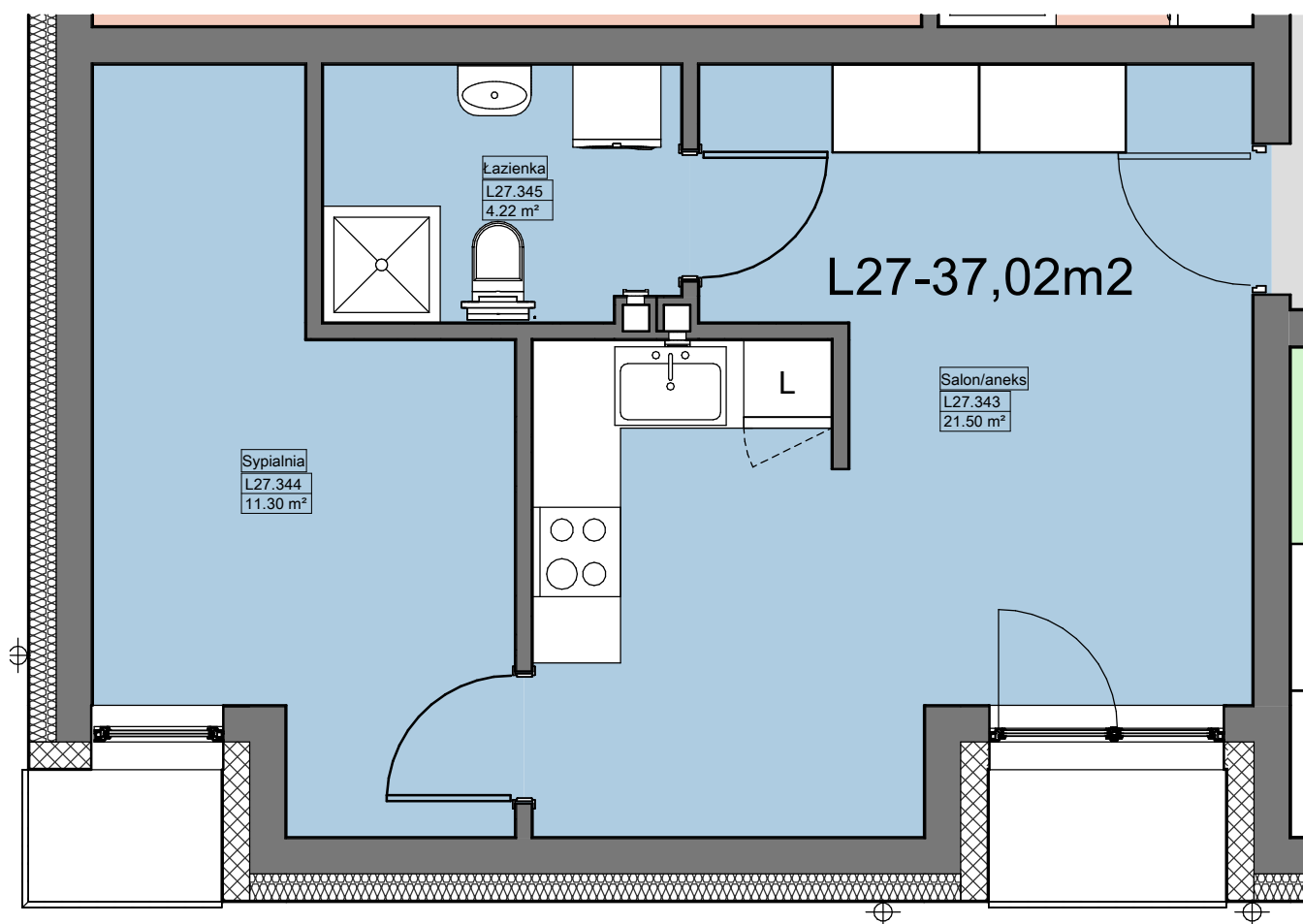
1 Rzut II Piętra — Lokal L27 1 : 50
