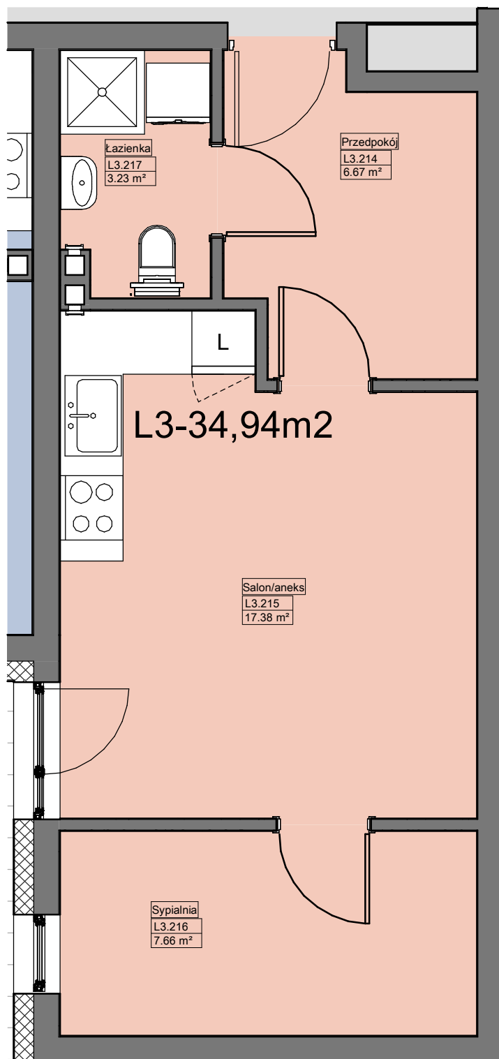
1 Rzut I Piętra — Lokal L3 1 : 50
