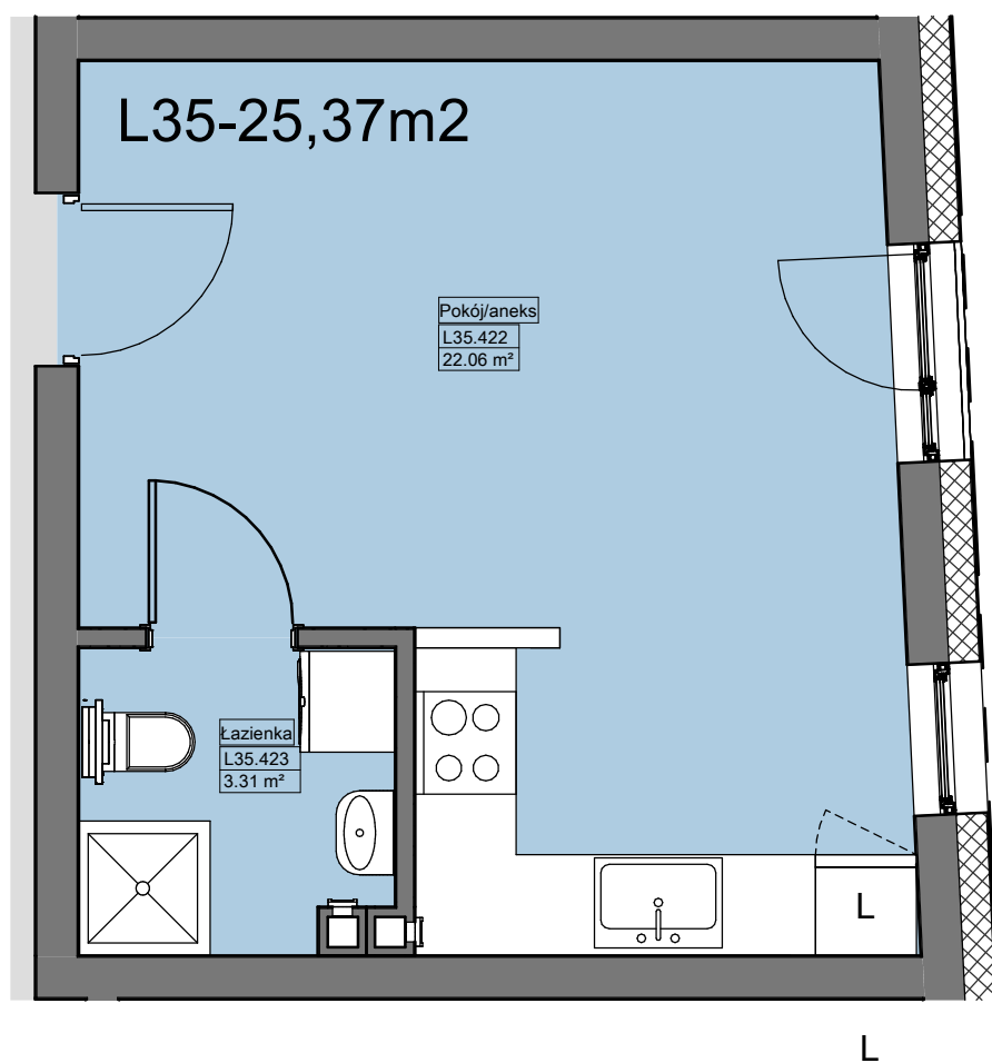
1 Rzut III Piętra — Lokal L35 1 : 50
