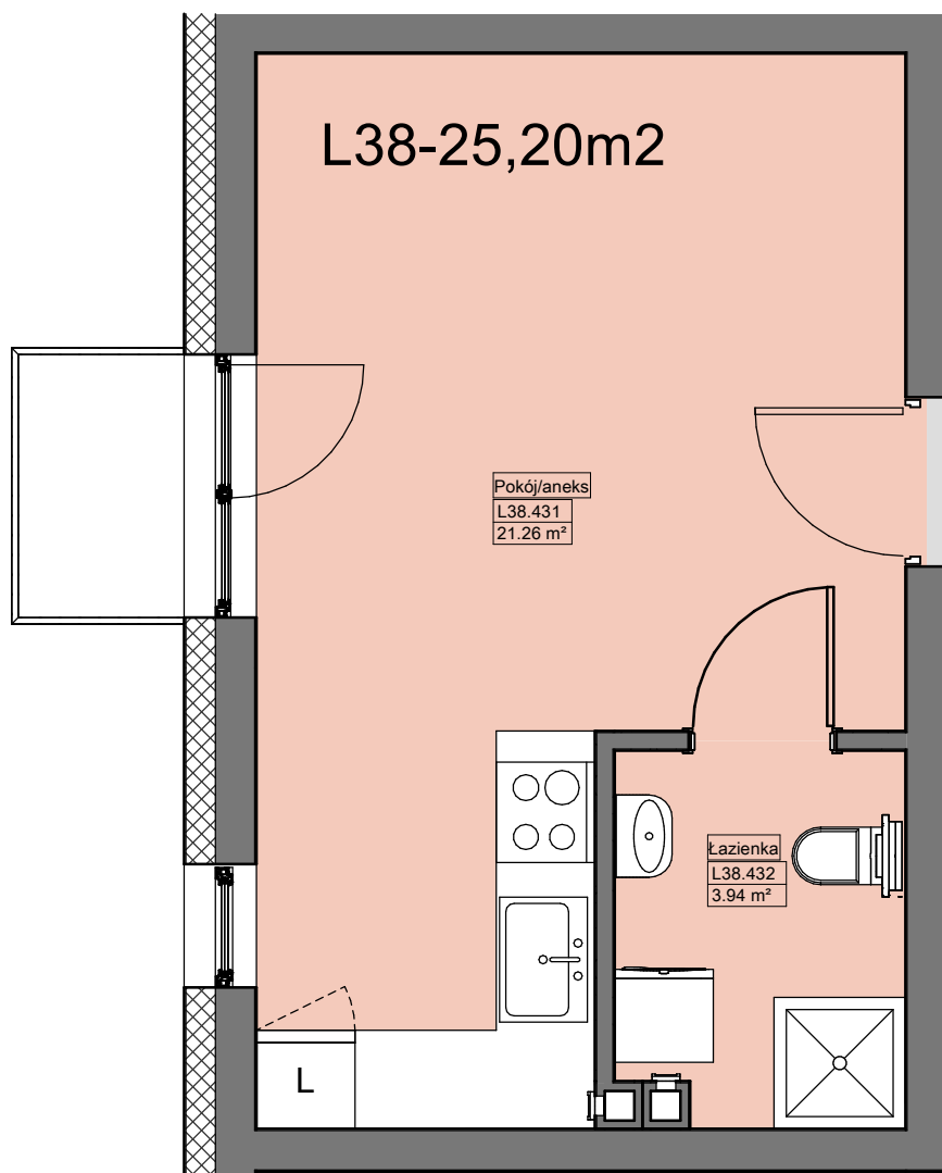
1 Rzut III Piętra — Lokal L38 1 : 50
