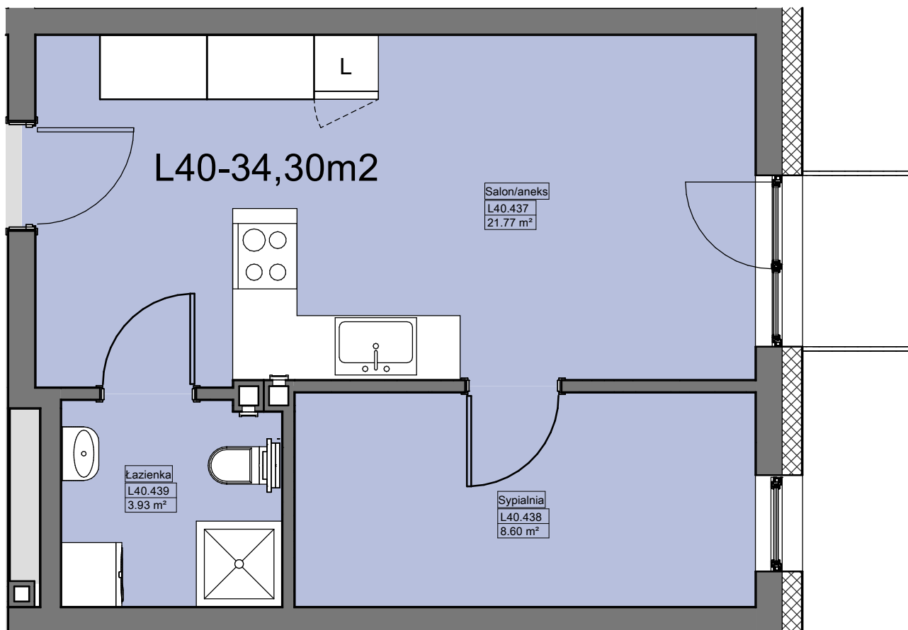
1 Rzut III Piętra — Lokal L40 1 : 50
