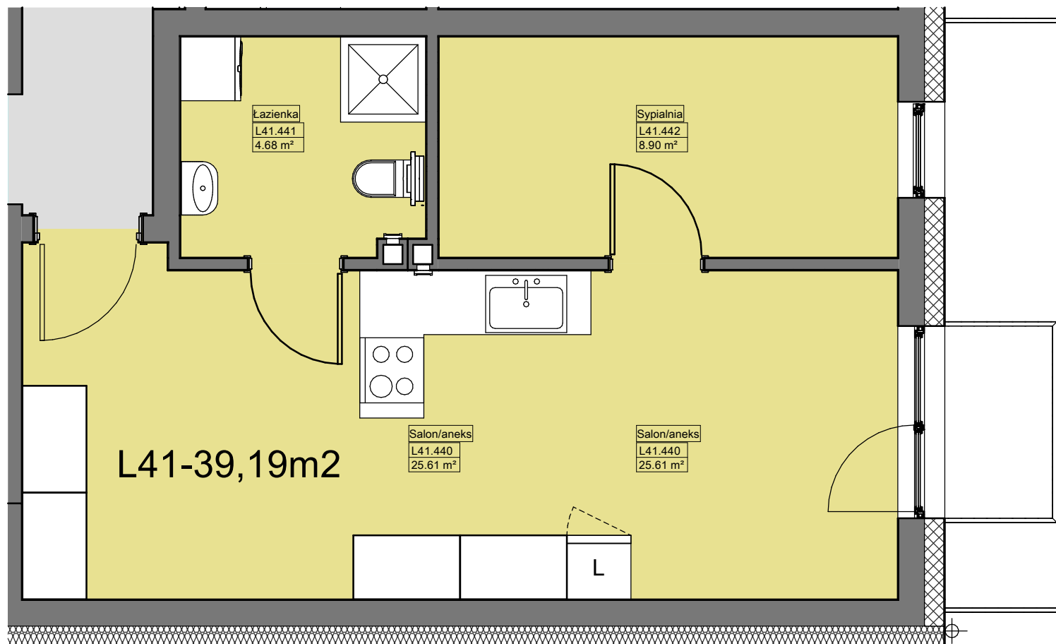
1 Rzut III Piętra — Lokal L41 1 : 50
