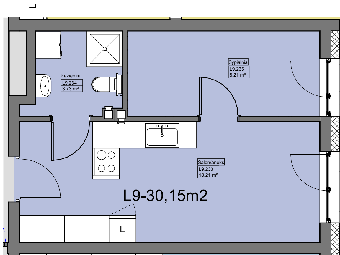
1 Rzut I Piętra — Lokal L9 1 : 50
